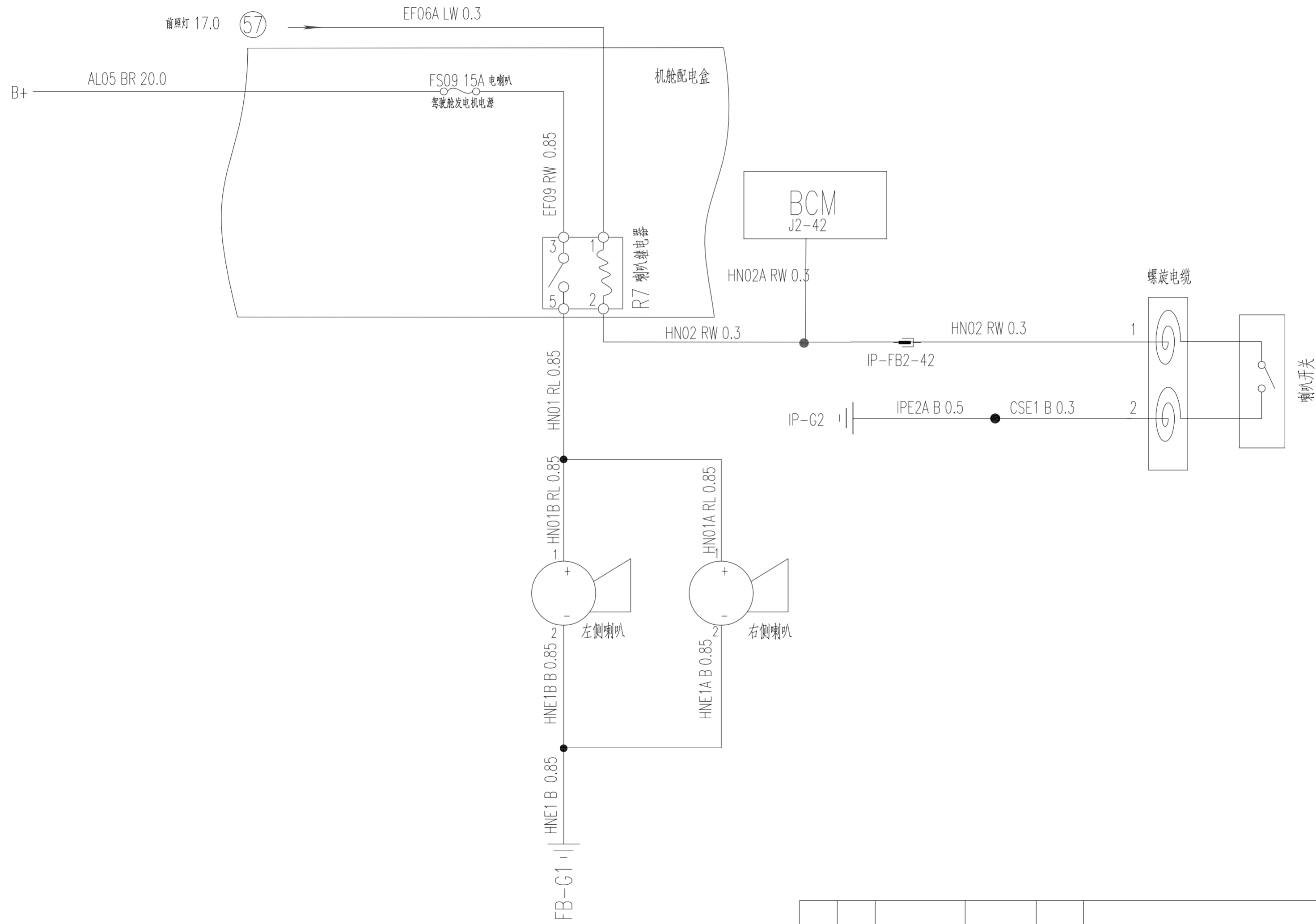
SX6A电气原理图
